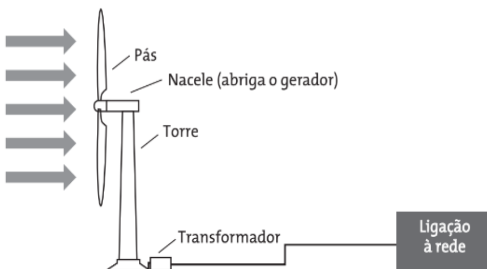
FIGURA 1 - COMPONENTES DE UM AEROGERADOR
